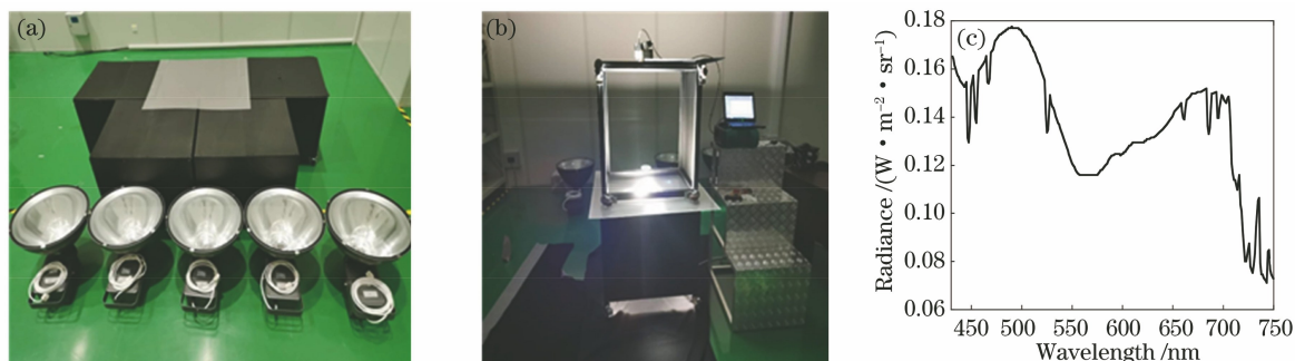
图 4 地面实验。(a)金属卤化物灯;(b)光源辐亮度测试现场;(c)光源辐亮度曲线
