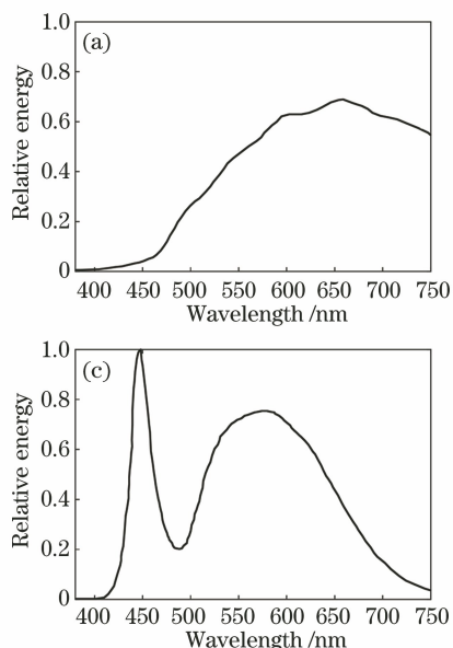
图 2 四种光源的光谱特性曲线。(a) 卤素灯; (b) 高压钠灯; (c) 发光二极管灯; (d) 荧光灯
