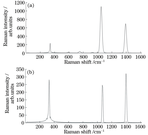
图 12 不同视场范围的光谱。(a) \pm 1.3^\circ ; (b) \pm 2.5^\circ Fig. 12 Spectra in different FOV ranges. (a) FOV of \pm 1.3^\circ ; (b) FOV of \pm 2.5^\circ
