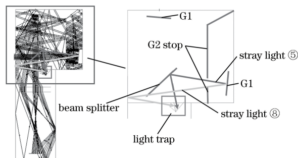
图 8 补偿漏光的光学陷阱的位置
