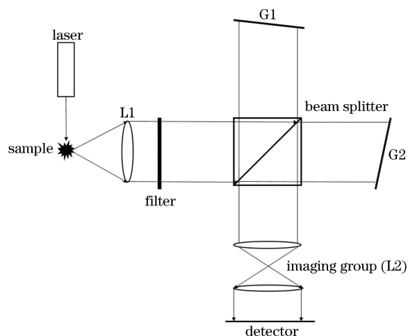
图 1 SHRS 的光学结构
