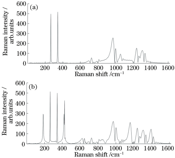
图 3 多波长噪声叠加。(a) 1120 nm 和 1130 nm 信号噪声; (b) 1110, 1120, 1130, 1140 nm 信号噪声
