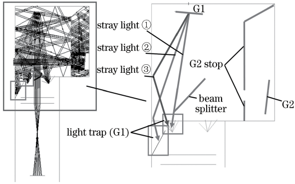
图 9 光学陷阱及挡板的位置 Fig. 9 Positions of light traps and baffles
