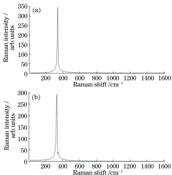
图 14 抑制后的多视场光谱。(a) \pm 1.3^\circ 视场; (b) \pm 2.5^\circ 视场
