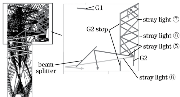
图 6 G2 光阑的位置
