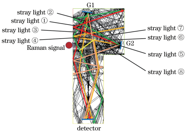
图 4 杂散光来源分布
