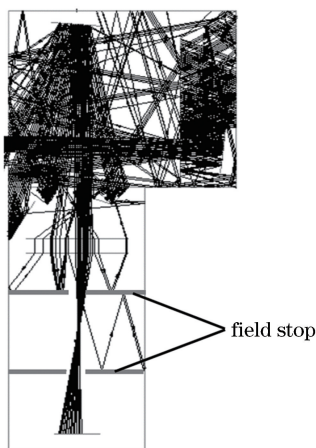
图 13 视场光阑示意图
