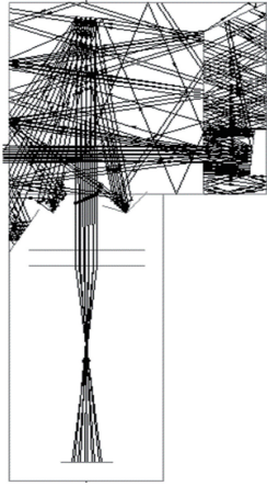
图 10 抑制杂散光后的系统光路图 Fig. 10 Light path after stray light control
