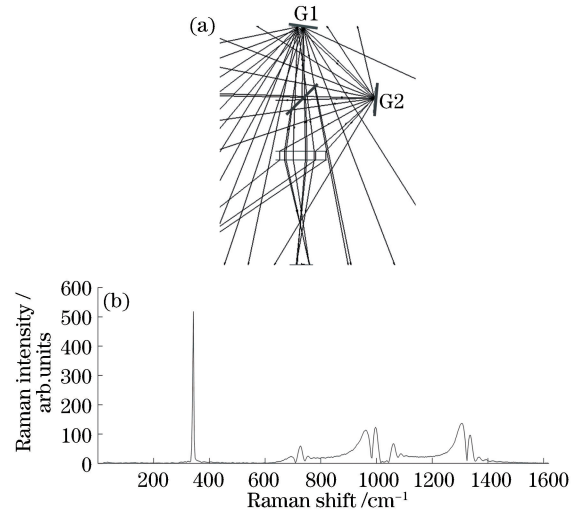
图 2 角度分布与拉曼光谱。(a)各级次角度分布; (b)单一波长多级衍射拉曼光谱
