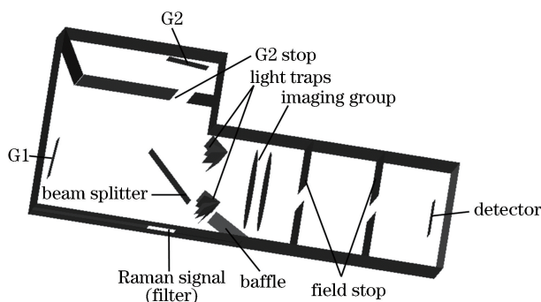
图 15 系统结构图
