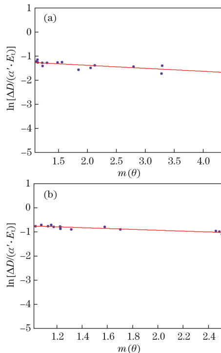
图 4 定标曲线拟合结果。(a) 2017 年 7 月 25 日; (b) 2017 年 8 月 30 日
