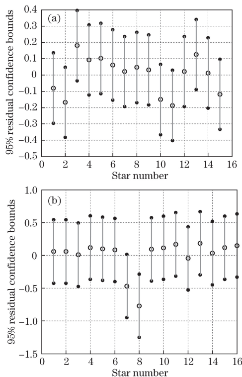
图 3 数据拟合的残差区间。(a) 2017 年 7 月 25 日; (b) 2017 年 8 月 30 日
