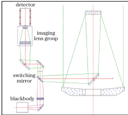
图 1 红外辐射测量系统的光学结构
