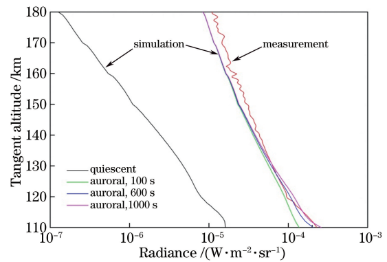
图 11 SABER 观测事件的模拟值与实测值对比
