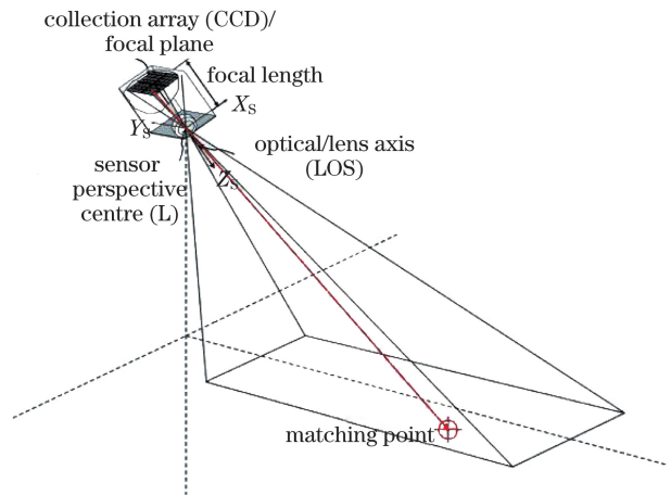
图 4 航空相机坐标系 Fig. 4 Schematic of aerial camera coordinate
