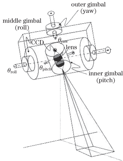
图 3 航空相机结构示意图 Fig. 3 Diagram of aerial camera
