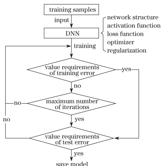
图 4 深度神经网络建模过程 Fig. 4 Modeling process of DNN
