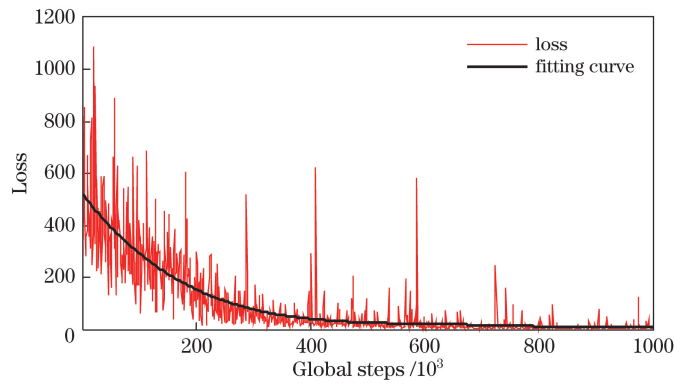
图 8 环氧漆损失函数数值下降曲线
