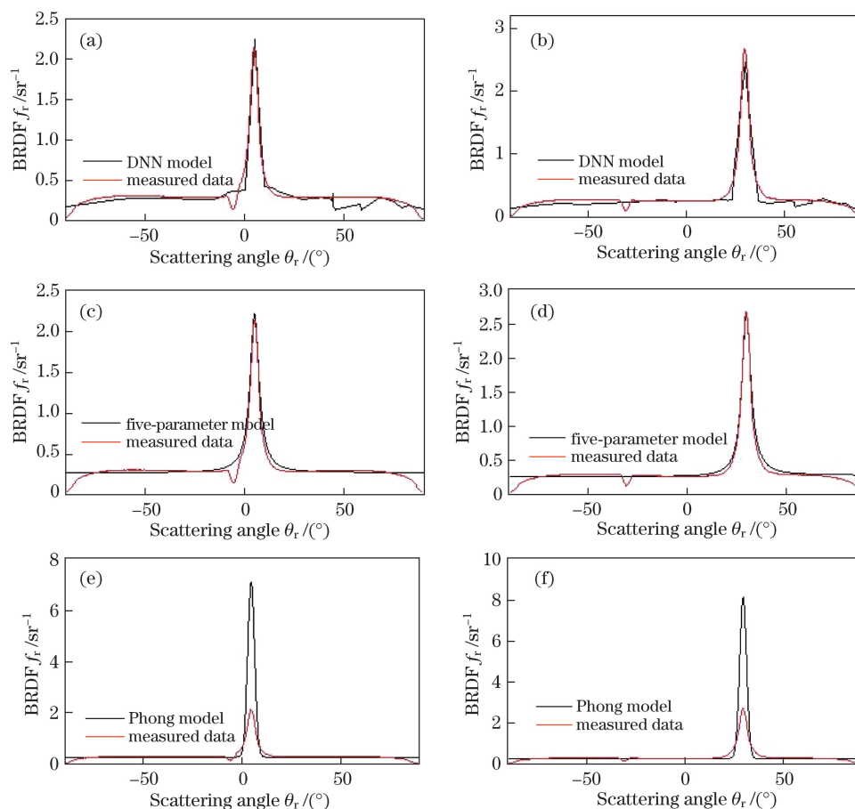
图 9 三种模型对环氧漆的拟合效果对比。神经网络模型: (a) \theta_i = 5^\circ , (b) \theta_i = 30^\circ ; 五参数模型: (c) \theta_i = 5^\circ , (d) \theta_i = 30^\circ ; Phong 模型: (e) \theta_i = 5^\circ , (f) \theta_i = 30^\circ
