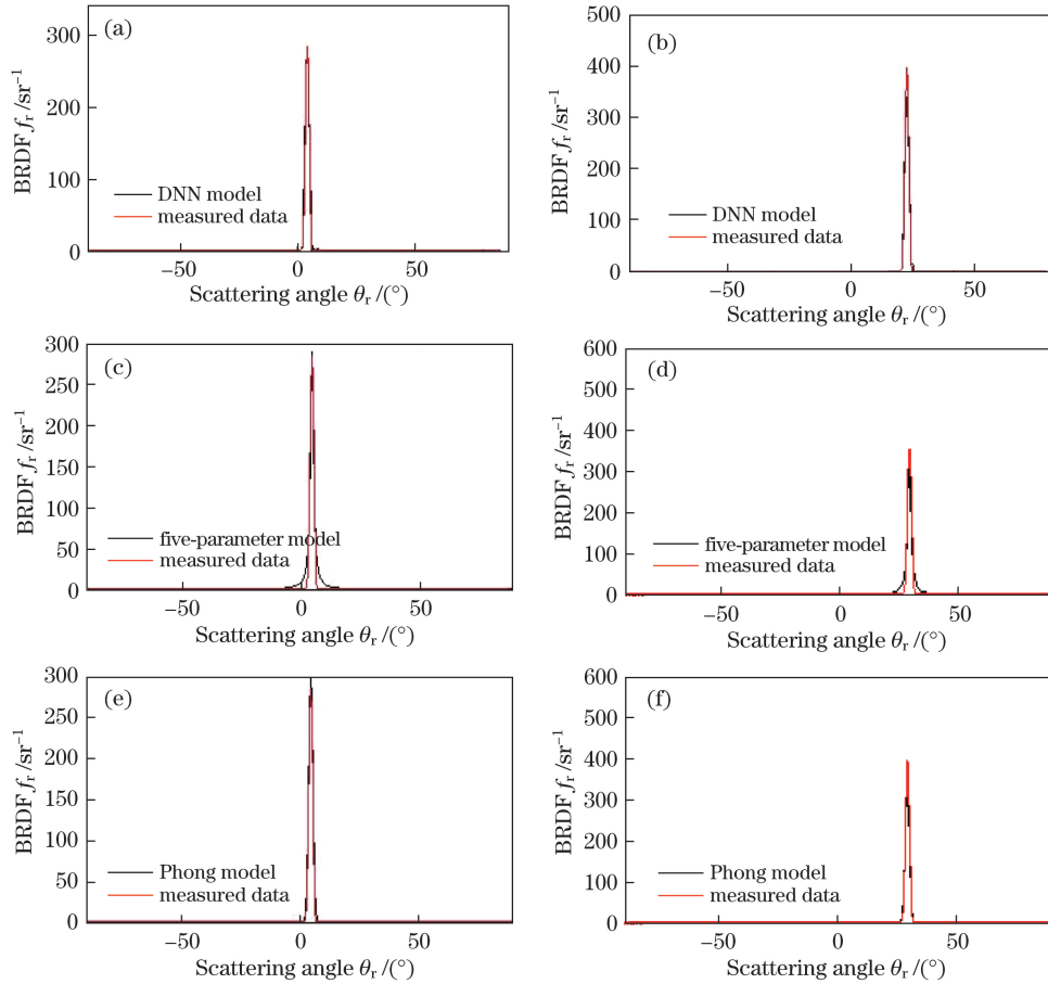
图 10 三种模型对聚酰亚胺薄膜的拟合效果对比。深度神经网络模型：(a) \theta_i=5^\circ ，(b) \theta_i=30^\circ ； 五参数模型：(c) \theta_i=5^\circ ，(d) \theta_i=30^\circ ；Phong 模型：(e) \theta_i=5^\circ ，(f) \theta_i=30^\circ
