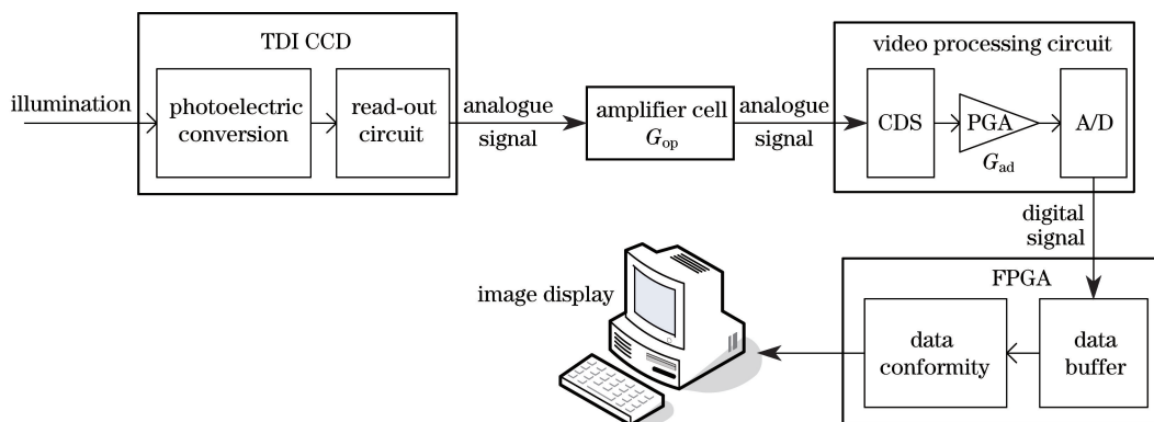
图 2 TDI CCD 成像系统信号处理流程
