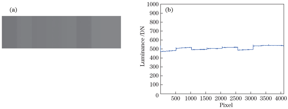
图 5 1/2 饱和时成像系统的响应输出。(a) 1/2 饱和时原始图像数据;(b) 1/2 饱和时灰度分布图 Fig. 5 Response output of imaging system under 1/2 saturation. (a) Raw image data of 1/2 saturation; (b) gray distribution of 1/2 saturation
