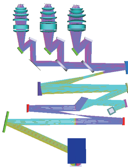
图 9 高光谱成像仪的光学结构图
