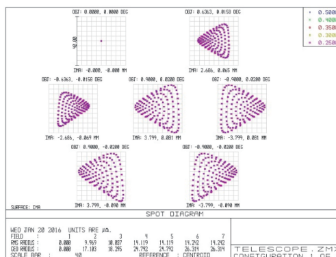
图 6 入射狭缝上的点列图分布
