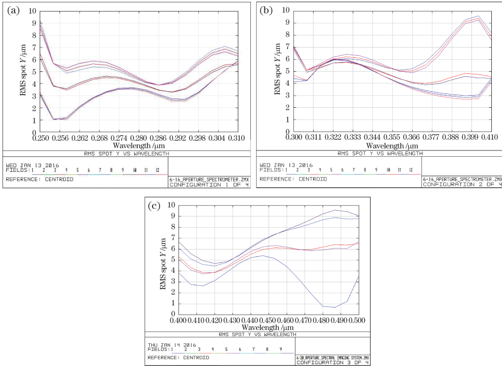
图 8 点列图均方根半径随波长的变化关系。(a)通道 1: 250~310 nm;(b)通道 2: 300~410 nm;(c)通道 3: 400~500 nm Fig. 8 RMS spot radius versus wavelength. (a) Channel 1: 250~310 nm; (b) channel 2: 300~410 nm; (c) channel 3: 400~500 nm
