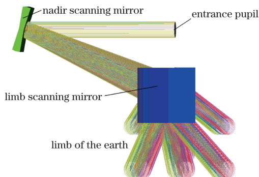
图 4 方位扫描镜扫描示意图
