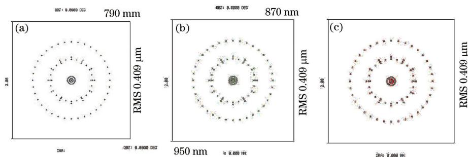
图 3 非球面透镜的像点图
