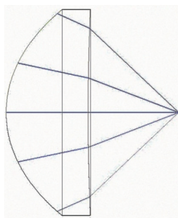
图 2 非球面透镜
