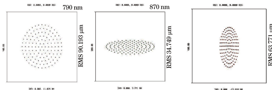
图9 光学系统的像点图
