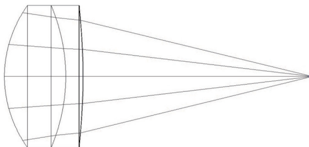
图4 透镜组
