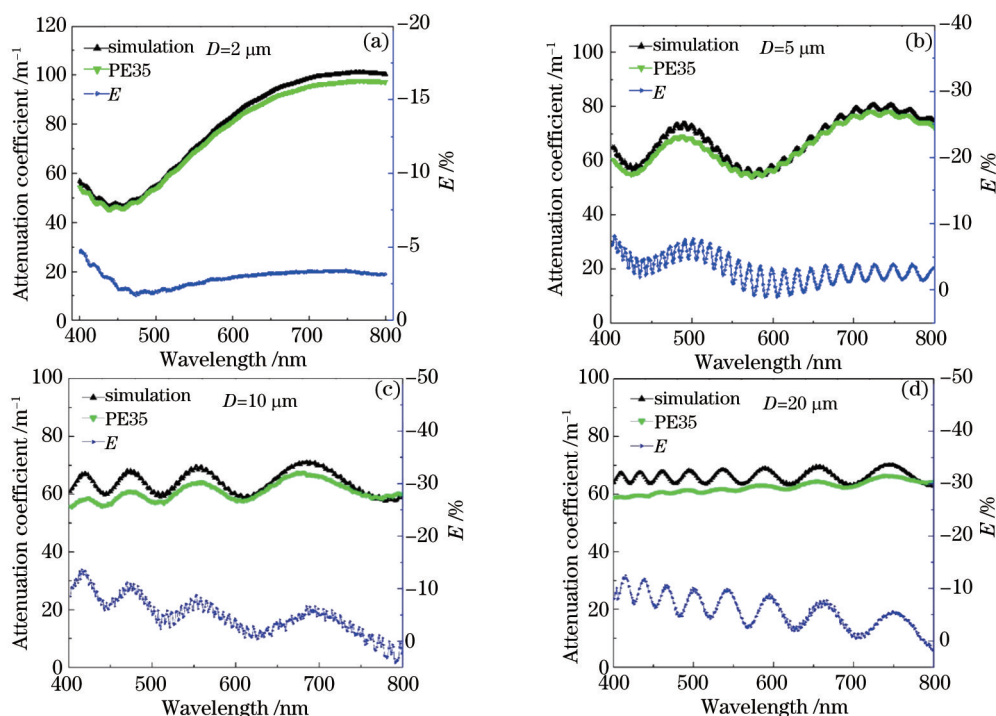
图 2 不同粒径标准颗粒的衰减系数测量值与理论计算值的比较(以标准颗粒的数量浓度归一化,单位为 \text{g}/\text{m}^3 )
