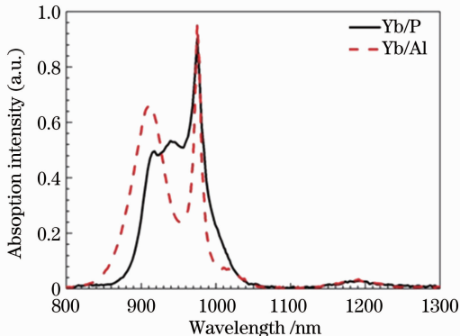
图 3 Yb/P 和 Yb/Al 光纤的吸收光谱
