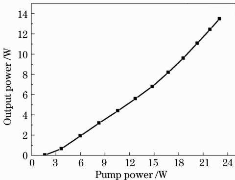
图 9 7 m Yb/P 光纤激光器输入输出关系
