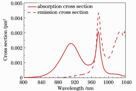
图 5 Yb/Al 光纤的吸收和发射截面
