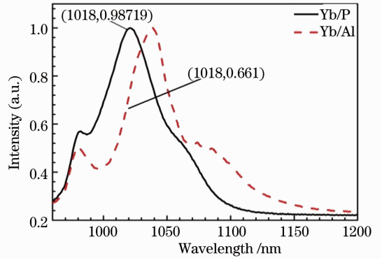
图 4 Yb/P 和 Yb/Al 光纤荧光光谱
