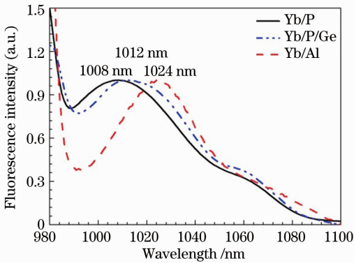
图 2 预制棒切片荧光次峰光谱
