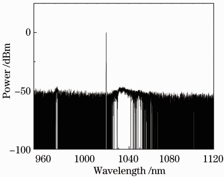
图 8 7 m 长增益光纤激光光谱
