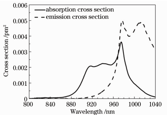
图 6 Yb/P 光纤的吸收和发射截面
