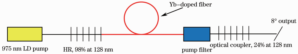
图 7 光纤激光测试示意图
