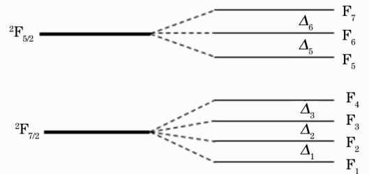
图 1 \text{Yb}^{3+} 精细结构能级
