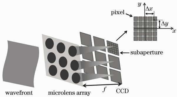
图 1 夏克-哈特曼波前传感器原理示意图 Fig. 1 Principle map of Shack-Hartmann wavefront sensor
