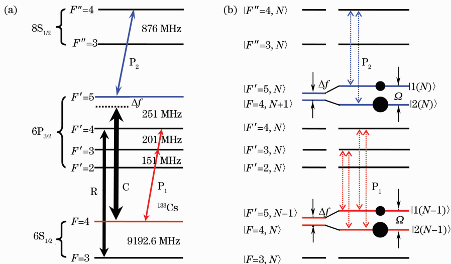
图 1 相关的铯原子超精细能级。(a)裸态;(b)缀饰态
