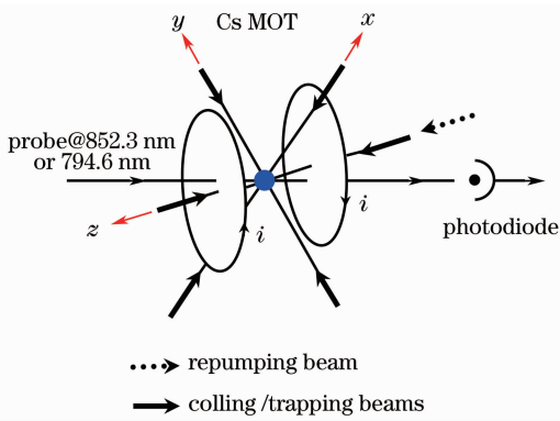
图2 实验装置示意图
