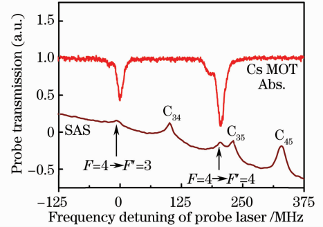
图3 冷原子中基态 6S_{1/2} F=4 \rightarrow 6P_{3/2} F'=3, 4 的缀饰态光谱
