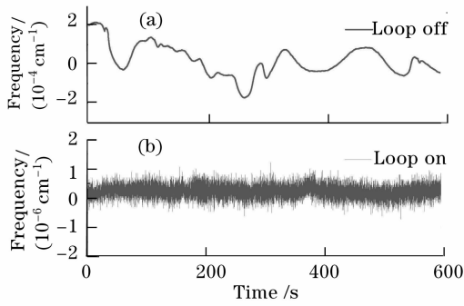
图4 EOM调制解调方法稳频时Nd:YAG激光器输出的频率稳定性
