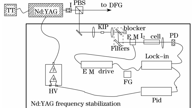
图 2 EOM 调制解调方法用于 Nd:YAG 激光稳频
