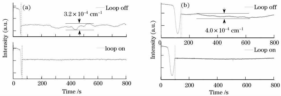
图 6 EOM (a)和 PZT(b)调制解调方法稳频 Nd:YAG 激光时 DFG 输出的频率稳定性
