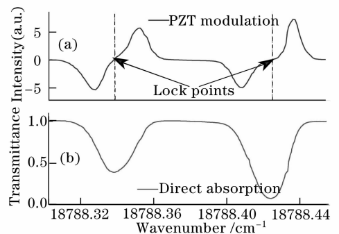
图 3 \text{I}_2 多普勒展宽直接吸收和调制解调谱
