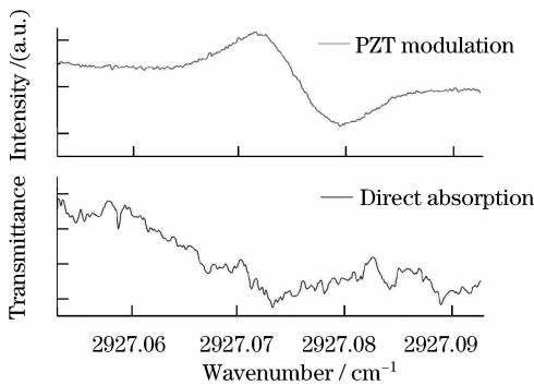
图 7 痕量 CH 4 在 2927.0762 cm -1 处的吸收线的直接吸收和 PZT 调制解调信号的比较
