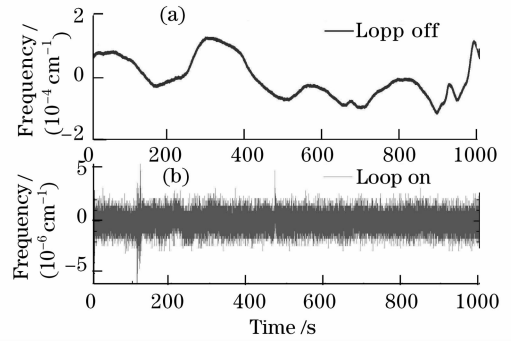
图5 PZT调制解调方法稳频时Nd:YAG激光器输出的频率稳定性
