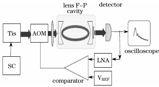
图 1 实验装置图: SC, 激光频率扫描控制系统; TiS, 钛宝石单模单频激光器; AOM, 声光调制器; LNA, 低噪声前置放大器; V_{REF} , 参考电压
