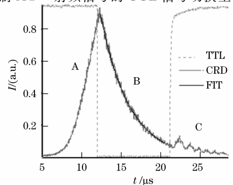
图 2 实验中观测到的透射的腔衰荡信号。其中, TTL 为迟滞比较电路输出控制声光调制器的触发信号、CRD 为透射的腔衰荡信号、FIT 为指数衰减理论拟合结果
