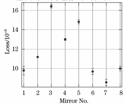
图3 8片超镜损耗测量结果
