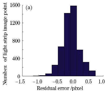
图 6 标定残差。(a)光平面 1 的标定残差；(b)光平面 2 的标定残差
