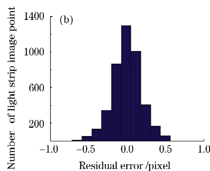
图 6 标定残差。(a)光平面 1 的标定残差；(b)光平面 2 的标定残差
