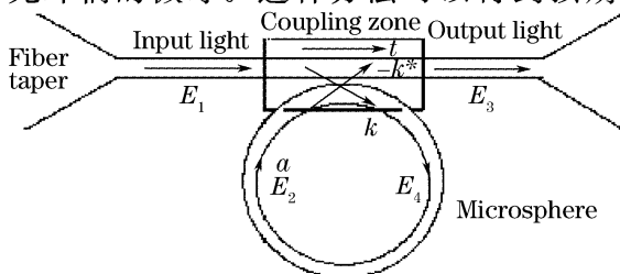
图 1 熔锥光纤与球微腔耦合系统示意图
