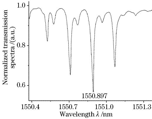
图 4 波长在 1550.897 nm 附近光谱的放大图
