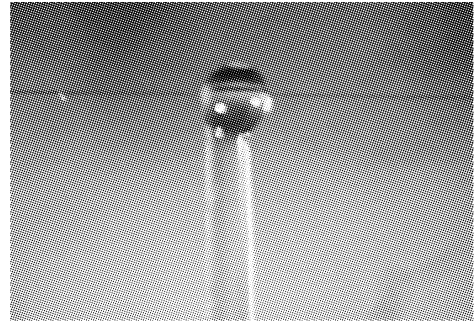
图 2 熔锥光纤与球微腔耦合系统实物图
