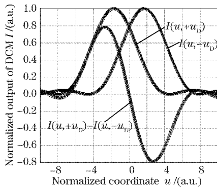
图 2 差动共焦输出信号
