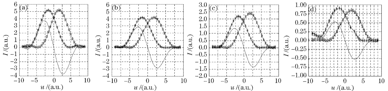
图6 差动共焦实验曲线。(a) 0°, (b) 10°, (c) 15°, (d) 18°
