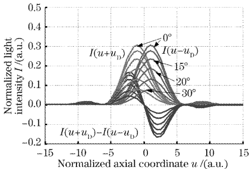
图 4 不同倾斜面的差动输出信号曲线
