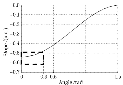
图 5 差动共焦输出曲线的零点处斜率
