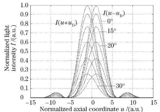
图 3 离焦时不同倾角的共焦轴向响应
