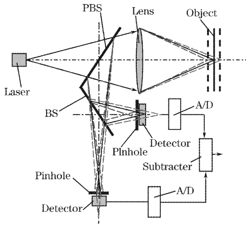
图 1 差动共焦原理图
