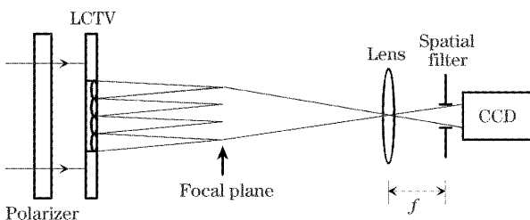
图 6 透镜阵列实验示意图 Fig. 6 The experimental setup for the lenslet array
