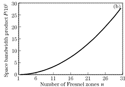
图 3 非涅耳带数与(a)焦距 f 和 F 数(b)空间带宽积的关系
