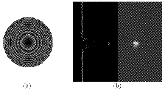
图 9 100 cm 焦距的连续相位透镜:(a)驱动函数,(b)测得的点扩展函数
