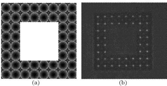
图 5 (a) 去掉中心 4 \times 4 阵列的 8 \times 8 阵列透镜和 (b) 光斑阵列
