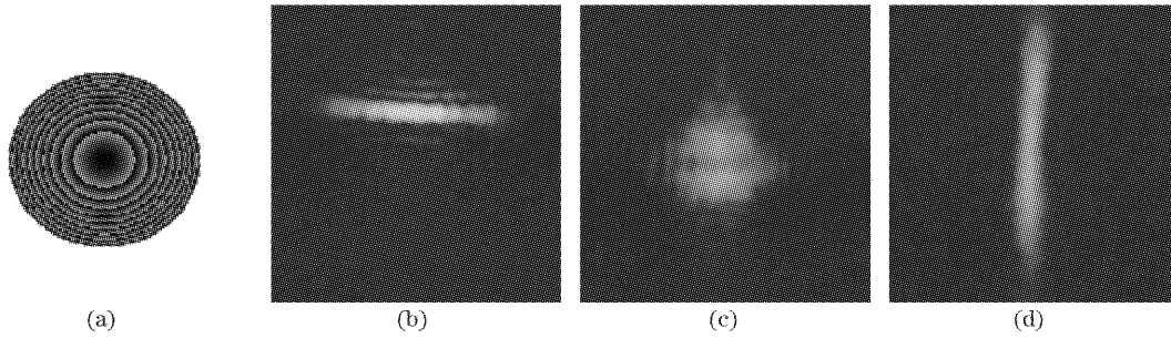
图 10 相位透镜
