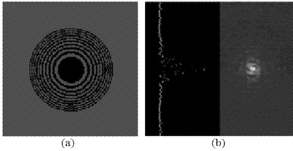
图 8 二进制相位透镜:(a)驱动函数,(b)测得的点扩展函数
