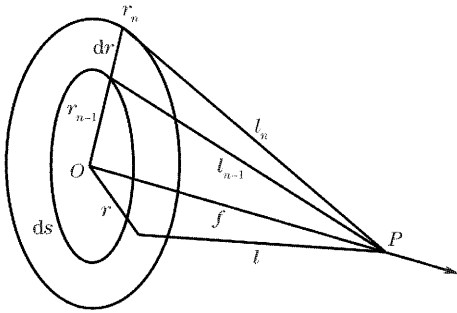
图 2 波前非涅耳带的焦点
