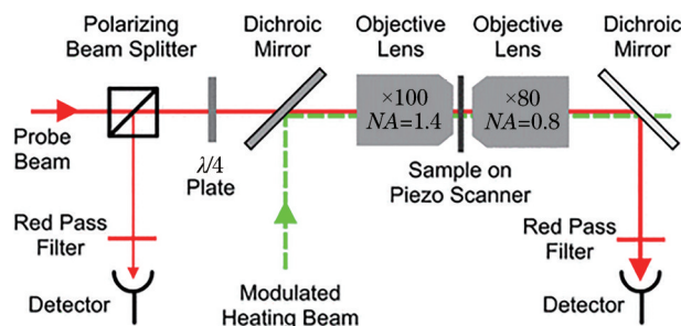
图 5 光热显微成像装置示意图 [31] (经许可转载,版权所有 2004,美国物理学会)
