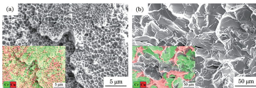
图 7 断口形貌和断面元素分布图。(a)熔凝层;(b)基体
