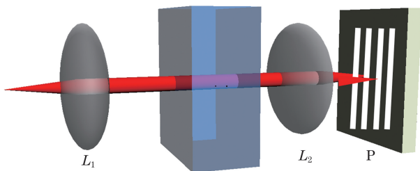
图 2 超声光栅的形成原理
