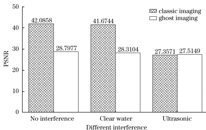
图 5 不同干扰条件下的 PSNR 柱状图
