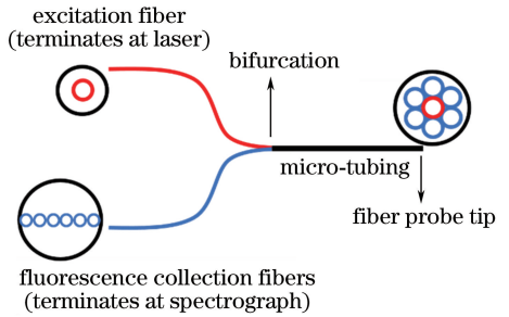
图1 典型的光纤荧光探针系统图
