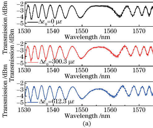
图 9 实验测量。(a) SFS 结构( L_{\text{FMF}} = 30 \text{ cm} )传输光谱随轴向应变变化;(b)特征波长随轴向应变的变化
