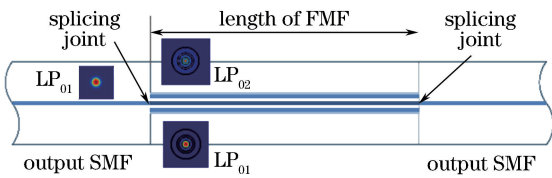
图 2 SFS 结构图
