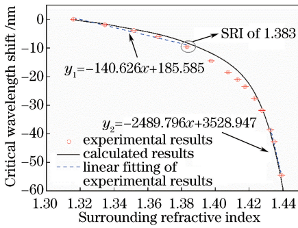
图 20 外界折射率变化下腐蚀 SFS 传输光谱中特征波长移动情况(实验结果标注误差线)
