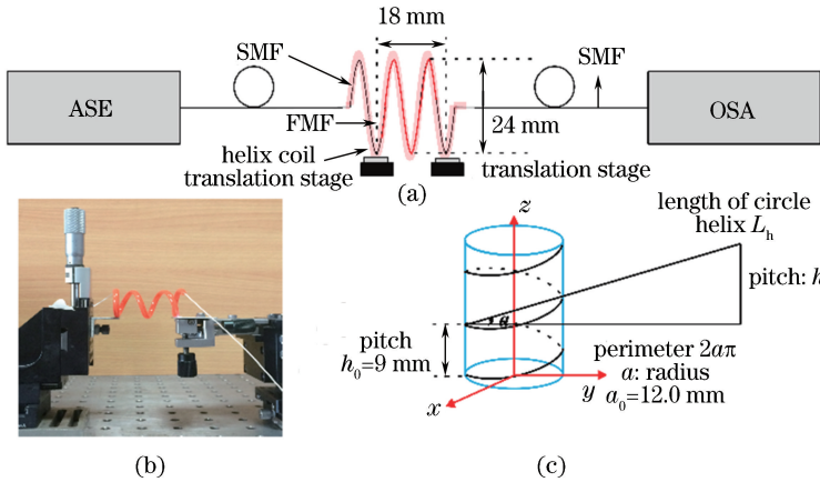
图 16 基于 SFS 结构 ( L_{FMF} = 10 cm) 的大量程位移传感器。(a) 实验示意图; (b) 实验实物图; (c) 螺旋管数学模型
