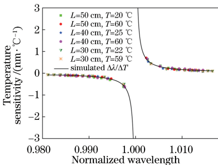
图 7 SFS 结构传输光谱中干涉条纹的温度灵敏度的仿真和实验曲线
