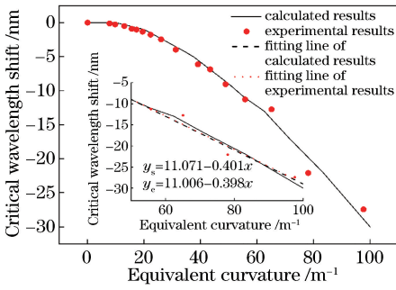
图 15 少模光纤的特征波长随等效曲率变化的仿真和实验结果
