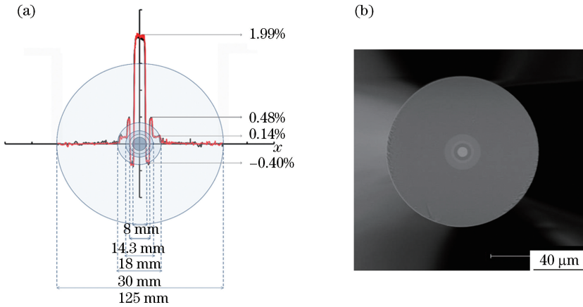
图 1 少模光纤横截面结构图。(a)几何示意图和归一化折射率差分布图;(b)扫描电镜图
