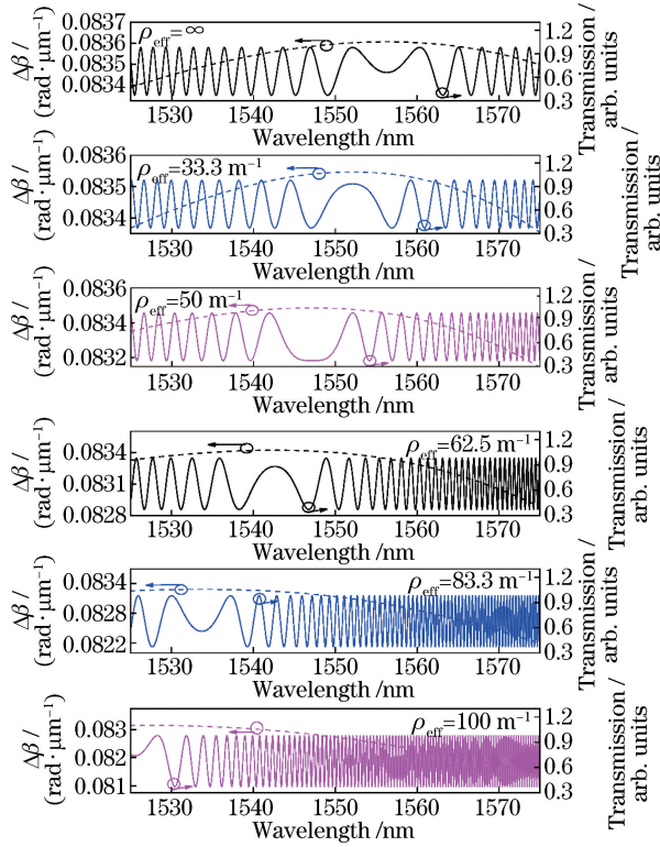
图 13 少模光纤在不同等效曲率下, 仿真 LP_{01} 模式和 LP_{02} 模式的 \Delta\beta 及 SFS 结构 ( L_{\text{FMF}} = 35 \text{ cm} ) 的传输光谱随波长的变化
