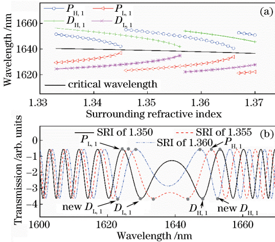
图 21 在外界折射率变化下,腐蚀 SFS 结构 ( d_{\text{FMF}} = 21.3 \mu\text{m} , L_{\text{FMF}} = 20 \text{ cm} ) 的传输光谱及特征波长和部分干涉峰/干涉谷波长的仿真变化。(a) 特征波长及左右两边干涉峰/谷 ( D_{\text{L},1} , P_{\text{L},1} , P_{\text{H},1} , D_{\text{H},1} ) 的波长移动情况;(b) SRI 为 1.350, 1.355, 1.360 时的传输光谱
