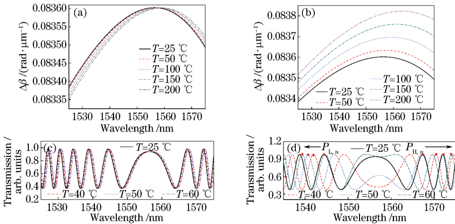
图 4 温度变化时, 少模光纤中传输的 \text{LP}_{01} 模式和 \text{LP}_{02} 模式的传播常数差 \Delta\beta 及 SFS 结构 ( L_{\text{FMF}} = 16 \text{ cm} ) 的传输光谱随波长变化的仿真曲线。(a) 不考虑热应力下的 \Delta\beta ; (b) 考虑热应力下的 \Delta\beta ; (c) 不考虑热应力下的传输光谱; (d) 考虑热应力下的传输光谱
