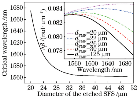
图 18 腐蚀 SFS 传输光谱中特征波长随光纤外径 d_{\text{FMF}} 变化的仿真曲线。其中插图为 \text{LP}_{01} 模式和 \text{LP}_{02} 模式的传播常数差在不同 d_{\text{FMF}} 下随波长变化的仿真曲线
