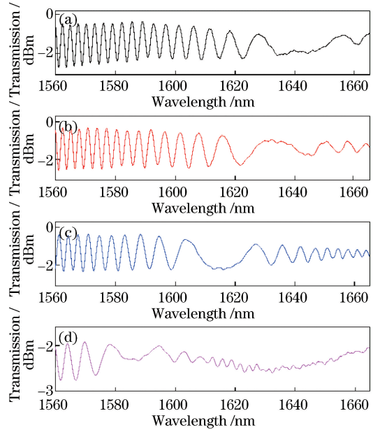
图 19 腐蚀 SFS 结构( L_{\text{FMF}} = 20 \text{ cm} , d_{\text{FMF}} = 21.3 \text{ μm} )在不同 SRI 下的传输光谱。(a) SRI 为 1.316; (b) SRI 为 1.383; (c) SRI 为 1.423; (d) SRI 为 1.439
