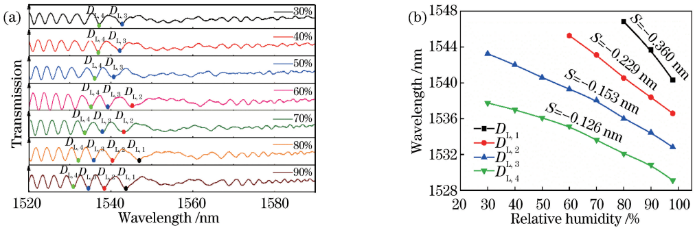
图 12 涂覆聚酰亚胺的 SFS 结构 ( L_{\text{FMF}} = 15 \text{ cm} ) 在相对湿度变化下的传感特性。(a) 传输光谱；(b) 干涉谷 D_{L,1}, D_{L,2}, D_{L,3}, D_{L,4} 的波长移动
