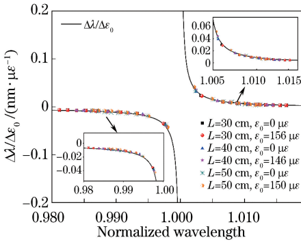
图 10 SFS 传感结构的传输光谱的干涉峰的轴向应变灵敏度随归一化波长的变化
