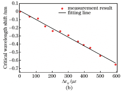
图 9 实验测量。(a) SFS 结构( L_{\text{FMF}} = 30 \text{ cm} )传输光谱随轴向应变变化;(b)特征波长随轴向应变的变化
