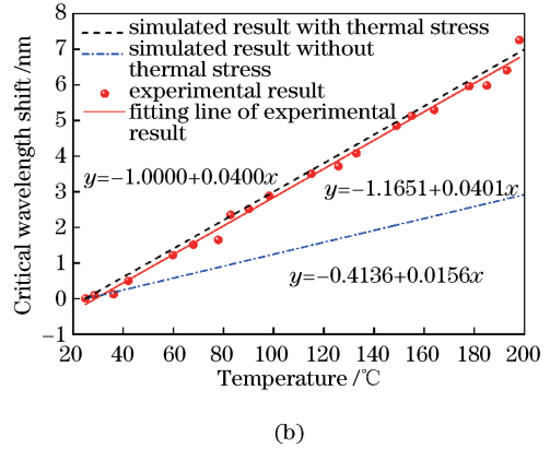
图 5 温度变化时 SFS 结构 ( L_{\text{FMF}} = 16 \text{ cm} ) 的实验传输光谱及特征波长的移动。
