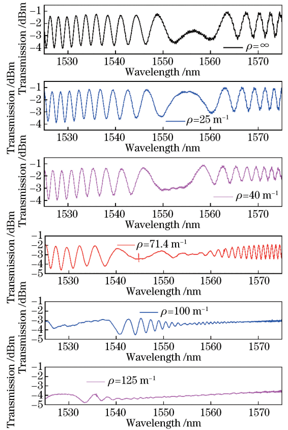
图 14 少模光纤在不同曲率下, 实验测得 SFS 结构 ( L_{\text{FMF}} = 35 \text{ cm} ) 的传输光谱随波长的变化
