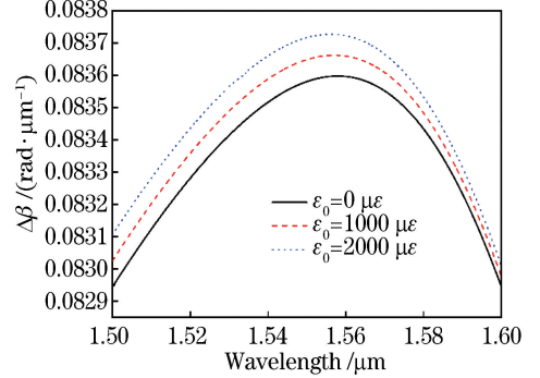
图 8 少模光纤中 LP 01 模式和 LP 02 模式之间传播常数差 \Delta\beta 随轴向应变变化的仿真曲线
