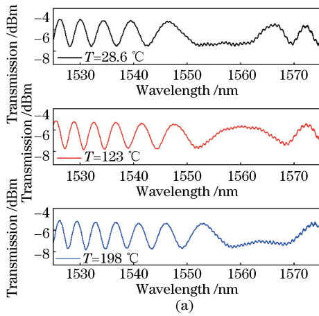
图 5 温度变化时 SFS 结构 ( L_{\text{FMF}} = 16 \text{ cm} ) 的实验传输光谱及特征波长的移动。
