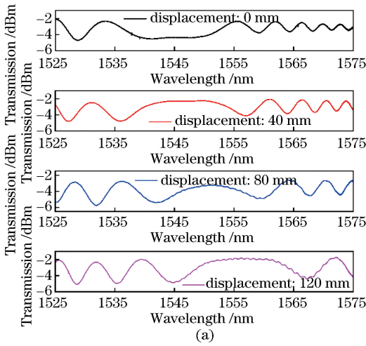
图 17 基于 SFS 结构( L_{\text{FMF}} = 10 \text{ cm} )的大位移传感器。(a)传输光谱随位移量的变化； (b)少模光纤等效曲率和特征波长随位移量的变化曲线
