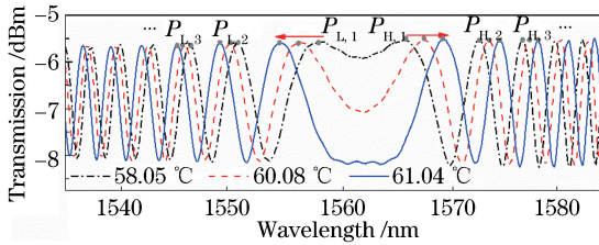
图 6 SFS 结构 ( L_{\text{FMF}} = 50 \text{ cm} ) 的传输光谱随温度的变化
