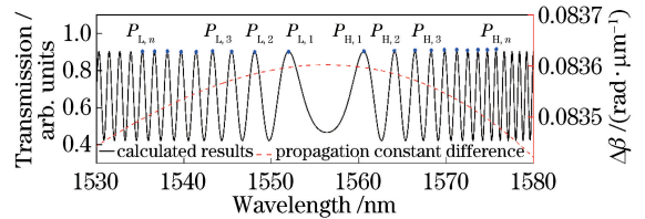
图 3 少模光纤中传输的 LP_{01} 模式和 LP_{02} 模式的传播常数差 \Delta\beta 和 SFS 结构 ( L_{FMF} = 50 cm) 传输光谱在 25 °C 自由状态下随波长变化的仿真曲线
