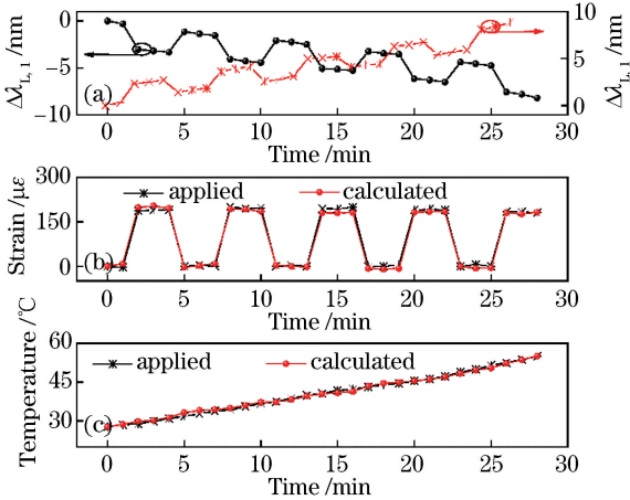
图 11 SFS 结构 ( L_{\text{FMF}} = 20 \text{ cm} ) 传感器随温度和轴向应变变化时的实时输出图。(a) 30 min 实验测试传输光谱中干涉峰 P_{H, 1} 和 P_{L, 1} 的峰值波长移动；(b) 实际施加轴向应力和 SFS 结构传感器实测输出轴向应力曲线；(c) 实际环境温度和 SFS 结构传感器实测输出温度曲线
