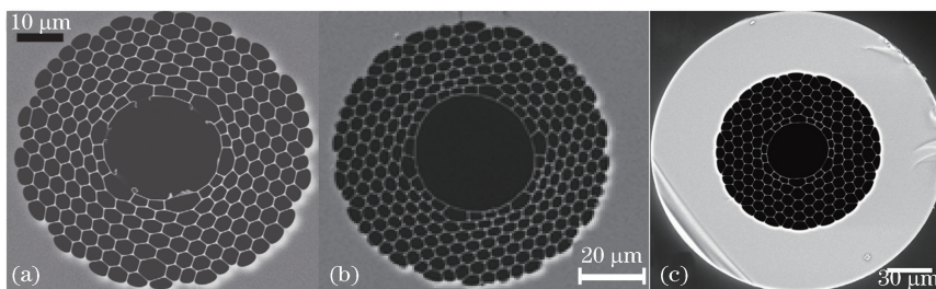
图 7 空芯光子带隙光纤。(a) 1.48 \text{ Tbit}/\text{s} 数据传输的空芯光子带隙光纤;(b) 73.7 \text{ Tbit}/\text{s} 数据传输的空芯光子带隙光纤;(c) 11 km 长的空芯光子带隙光纤
