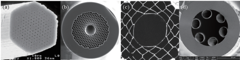
图2 不同导光机理的光子晶体光纤。(a)折射率导光型光子晶体光纤;(b)光子带隙光纤; (c)反谐振导光光纤;(d)单层无节点反谐振光纤
