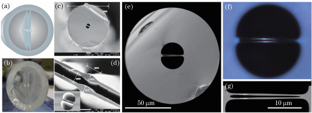
图8 双芯纳米机械光纤。(a)~(d)南安普顿大学的双芯光纤;(e)~(g)德国马克斯普朗克研究所的双平行玻璃片光纤
