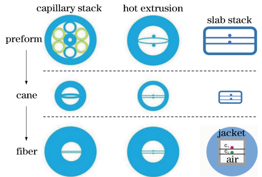
图9 纳米机械光纤预制棒制备方案
