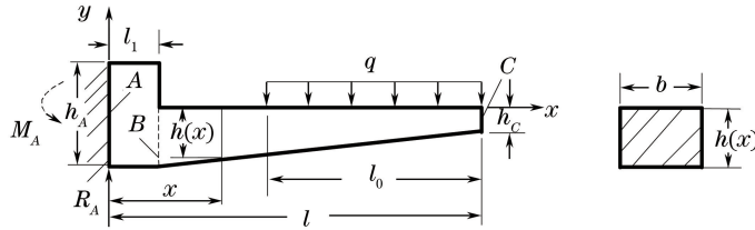
图4 升降平台计算模型
