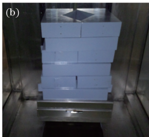
图 7 (a)升降平台样件;(b)载荷测试;(c)安装实验
