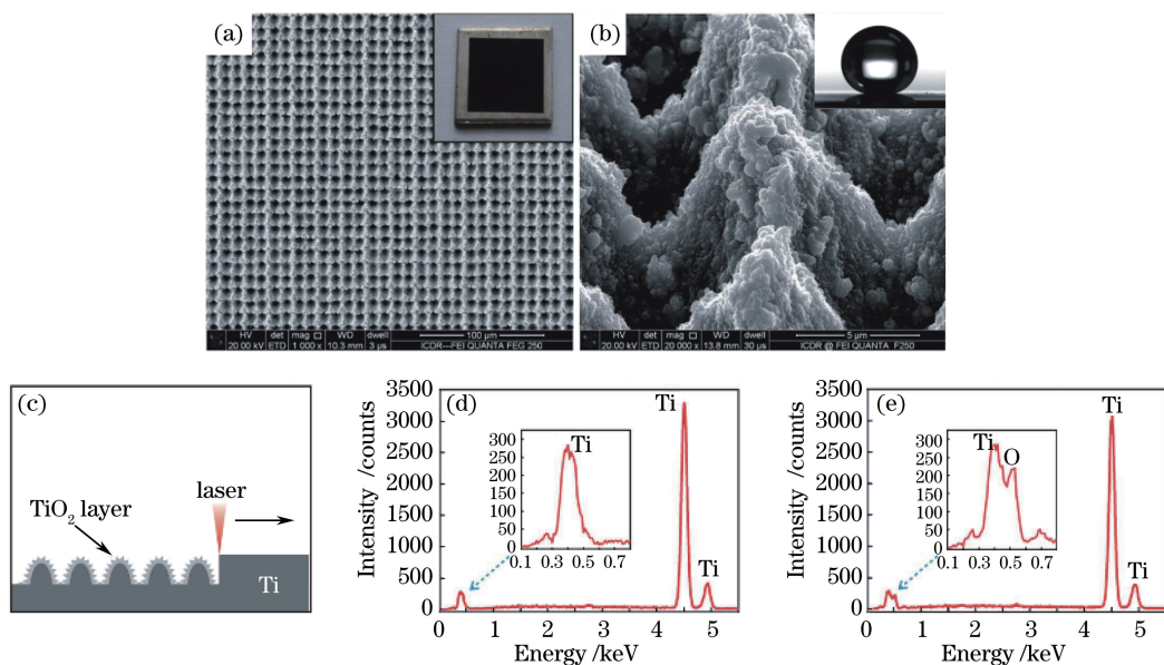
图 7 飞秒激光作用钛表面。(a)飞秒激光作用钛表面后的微观电镜图;(b)更高放大倍数的电镜图, 右上角为水滴的接触角投影图;(c)激光加工示意图;(d)激光扫描前和(e)激光扫描后的 EDXS 能谱 [89]
