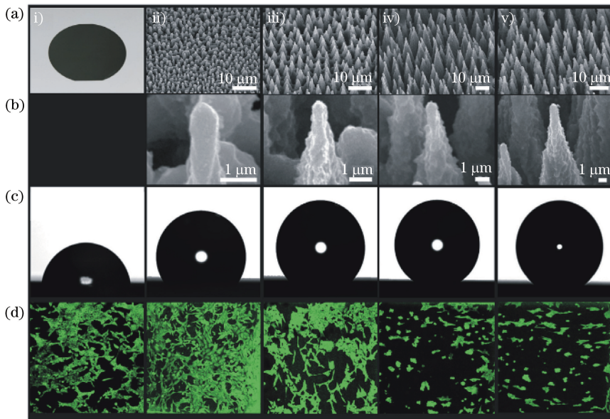
图 14 利用飞秒激光微加工技术调控活体细胞与生物材料间的相互作用。(a)平滑未加工情况及飞秒激光能量密度为 0.34,0.56,0.9,1.69 J/cm 2 时烧蚀出的硅微结构电镜图;(b)更高的电镜放大倍数;(c)水滴在不同样品上的投影形貌;(d)培养 3 d 后成纤维细胞染色的激光共聚焦显微镜图 [136]
