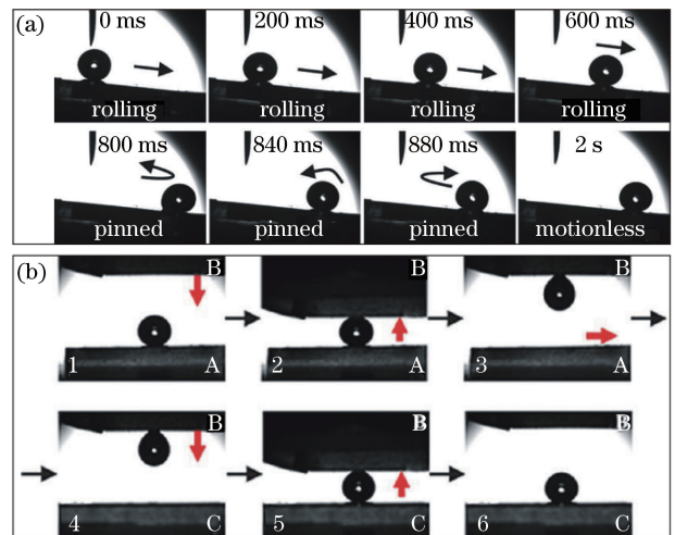
图 13 飞秒激光实现微液滴操控示意图。
