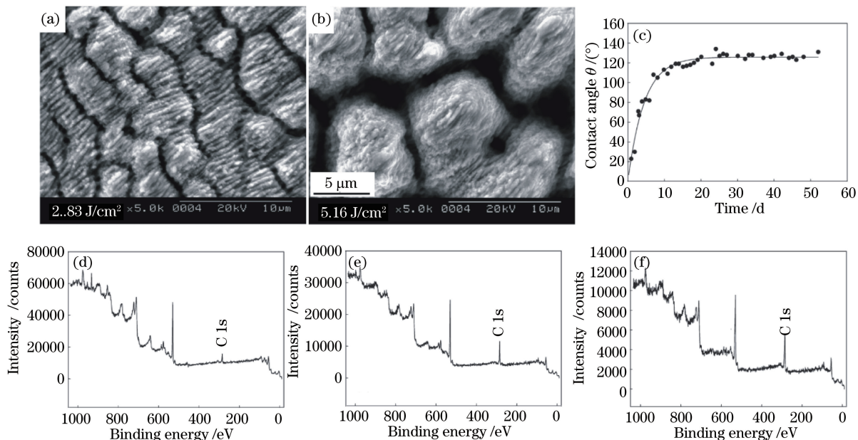
图 6 飞秒激光扫描不锈钢。功率密度为(a) 2.83 J/cm 2 和(b) 5.16 J/cm 2 的飞秒激光扫描不锈钢后的电镜图;(c)样品接触角与放置时间的关系图;(d)本征不锈钢的和(e)激光扫描后不锈钢的及(f)空气中放置 52 d 后的不锈钢的 XPS 能谱 [92]
