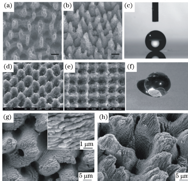
图 4 利用飞秒激光和表面硅烷化处理共同构建的超疏水粗糙表面。在六氟化硫气体中飞秒激光作用于硅片 [51] 的(a)俯视图, (b) 45^\circ 镜侧视图和(c)水滴的接触角投影图;在空气中飞秒激光作用于硅片 [72] 的(d) 45^\circ 侧视图, (e)俯视图和(f)水滴在硅片上的形貌图;在真空环境中飞秒激光作用于不锈钢 [69] 的(g)俯视图和(h) 45^\circ 镜侧视图
