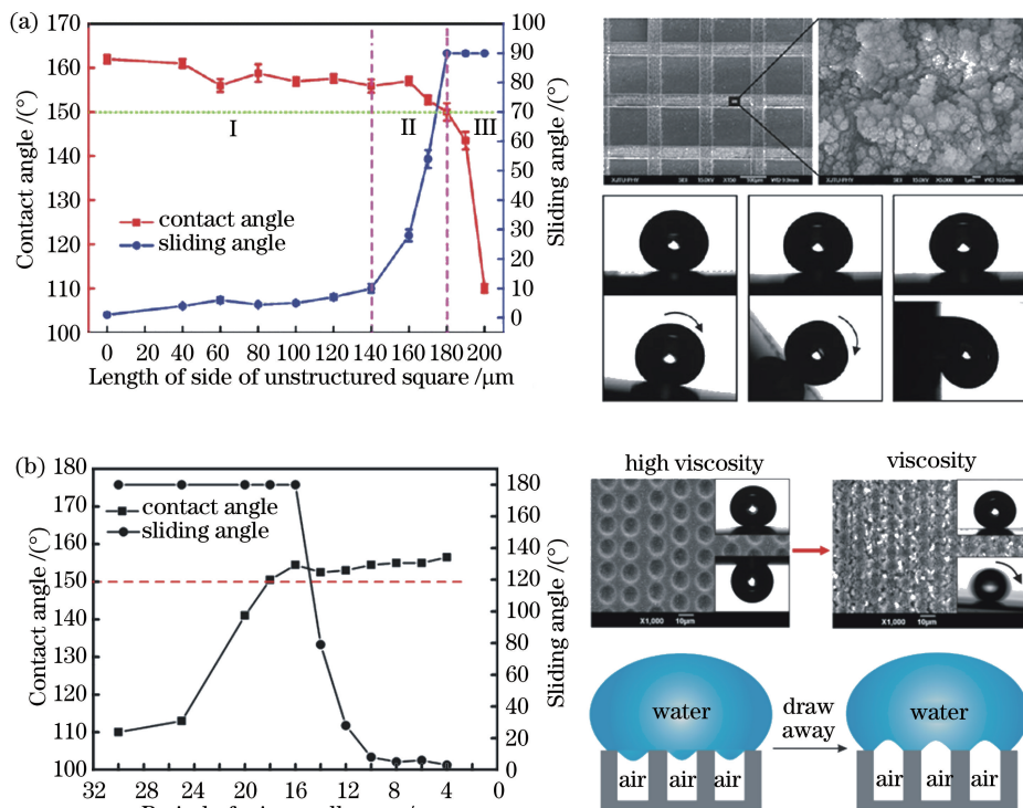
图 8 改变超疏水材料黏滞性的方法。(a)调控 PDMS 的井字形阵列间距 [87] ; (b)调控 PDMS 的脉冲烧蚀间距 [102]
