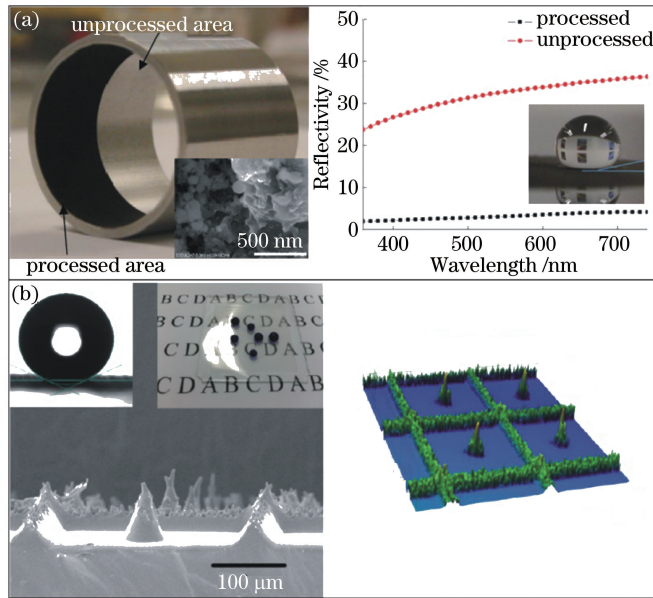
图 11 高光吸收率超疏水金属的制备。(a)飞秒激光扫描后金属材料表面的光吸收与超疏水特性 [117] ;
