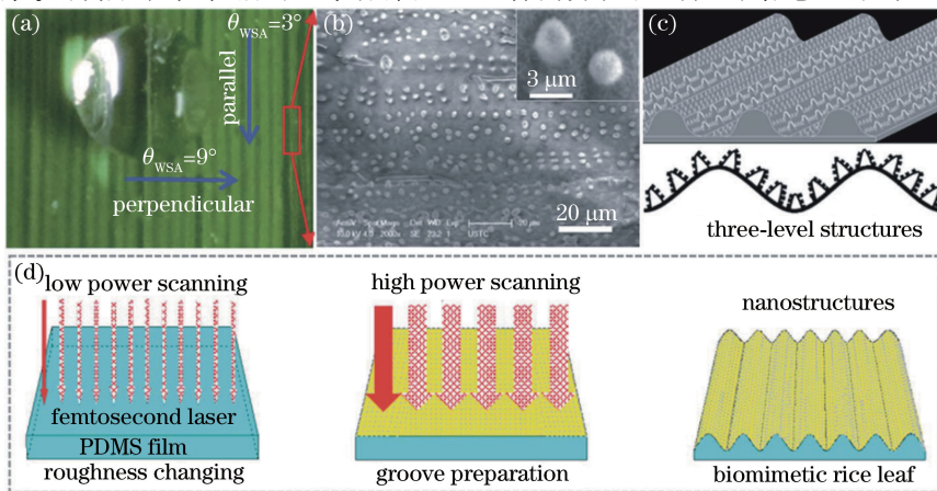
图 9 水稻叶的分级粗糙结构。(a) 水稻叶表面及其各向异性水滴滚动特性; (b) 水稻叶表面的俯视图电镜图; (c) 水稻叶的分级粗糙结构模型; (d) 飞秒激光制造仿水稻叶的原理示意图
