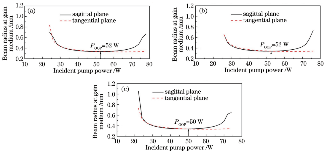
图 3 腔镜曲率半径和腔长均变化时,增益晶体处的基模束腰半径与抽运功率的关系。
