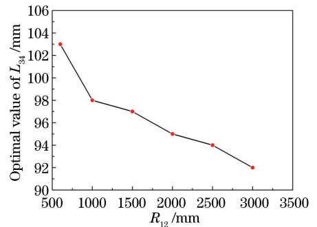
图 6 不同曲率半径下的最佳腔长 L_{34}
