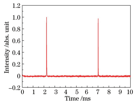
图 8 F-P 干涉仪扫描获得的激光器单频特性
