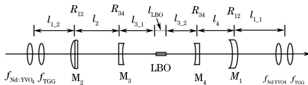
图 1 环形腔的等效薄透镜序列
