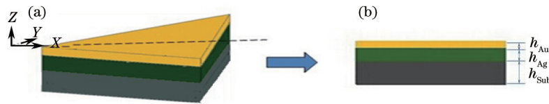
图 1 金银复合三角形纳米粒子的示意图。(a) 三维示意图; (b) 横截面图
