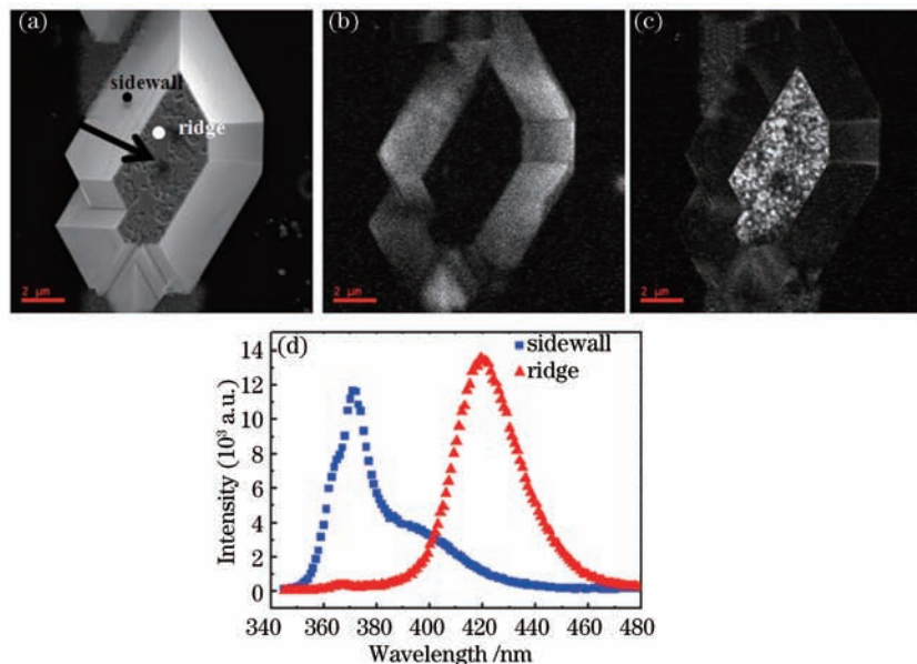
图 3 (a) GaN 半极性面生长 InGaN/GaN 多量子阱平面 SEM 图;(b) SEM 对应区域的 390 nm 单色 CL 谱;(c) SEM 对应区域的 420 nm 单色 CL 谱;(d) GaN 面上 InGaN/GaN 多量子阱斜面和顶点的局域点 CL 谱
