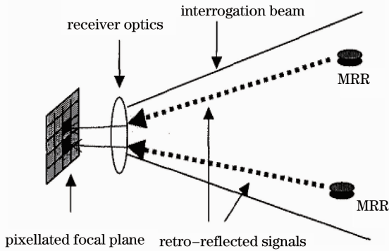
图 9 MRR 单元结构
