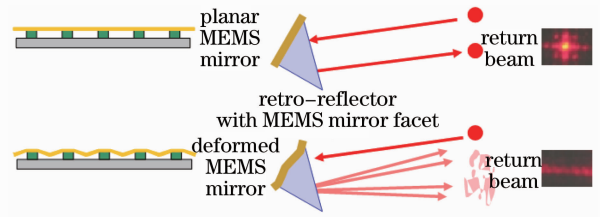
图 3 利用 MEMS 构建的 MRR FSO 链路及逆向调制器
