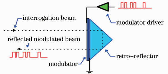
图 2 MRR 原理图
