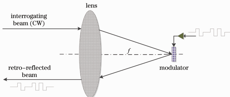
图 4 CE MRR 结构图
