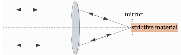
图 5 离焦型 MRR 结构图
