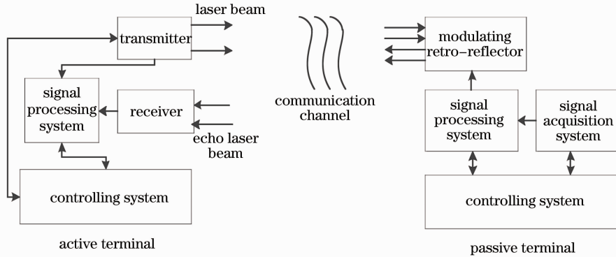
图 1 MRR FOS 系统结构图
