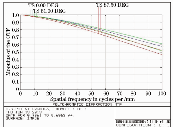
图 4 系统传递函数
