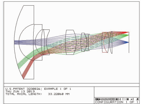
图 2 镜头系统结构
