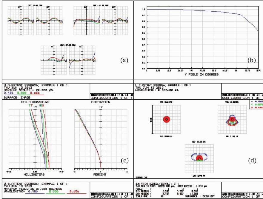
图 3 (a) 垂轴像差; (b) 相对照度; (c) 场曲畸变图; (d) 点列图
