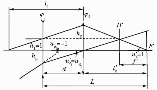
图 1 反远距型光学结构图
