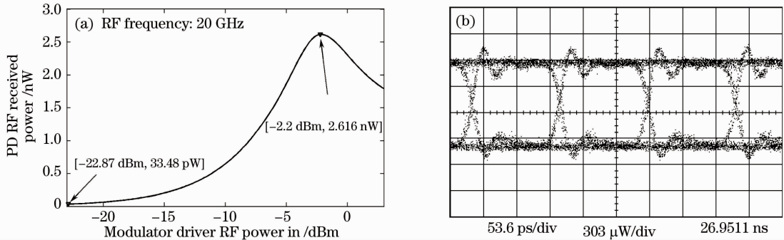
图 4 (a) 功率扫描, (b) 眼图测试
