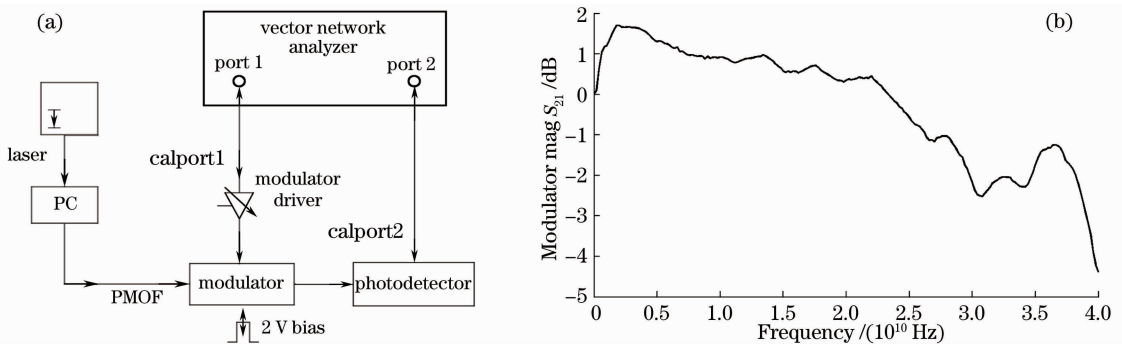
图 2 (a) 40 GHz 高速性能测试系统, (b) 去除误差后的光调制器 S_{21} 参数,其-3 dB 带宽为 34 GHz
