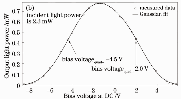
图 3 (a) 调制曲线测试系统, (b) 测试得到的调制曲线及其拟合曲线
