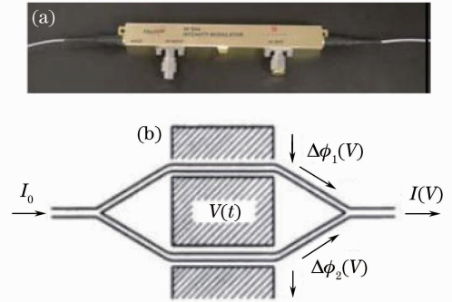
图 1 (a) Mach-40-005 40 GHz 调制器,
