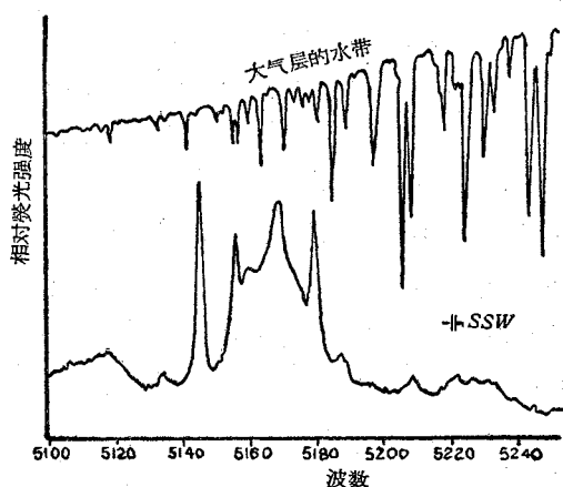
图 1 下面轨迹: 77°K, 含 1/2 原子% Tm 3+ 的 Er 2 O 3 中的 3 H 4 → 3 H 6 荧光光谱的一部分; 上面轨迹: 5,332 厘米 -1 水蒸汽带的 b 支。
