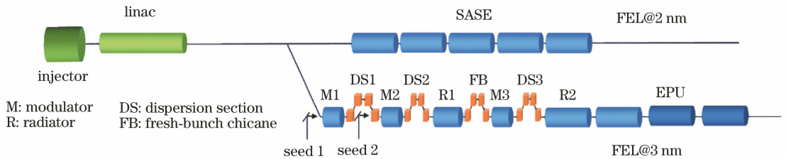
图 1 SXFEL-UF 布局示意图
