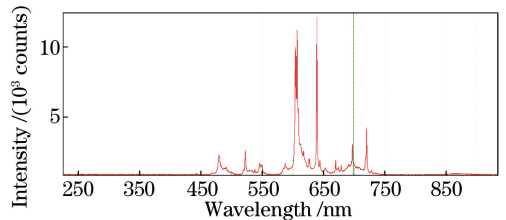
图 4 Pr:YLF 晶体的荧光谱线
