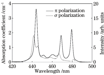
图 2 Pr:YLF 晶体偏振吸收谱
