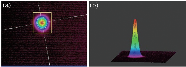
图 6 348.9 nm 紫外光轮廓。(a)二维成像图;(b)三维成像图
