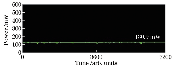
图 8 348.9 nm 激光器功率稳定性
