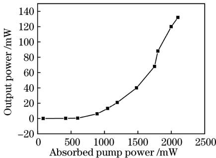
图 7 348.9 nm 激光的输出功率随吸收的抽运功率的变化
