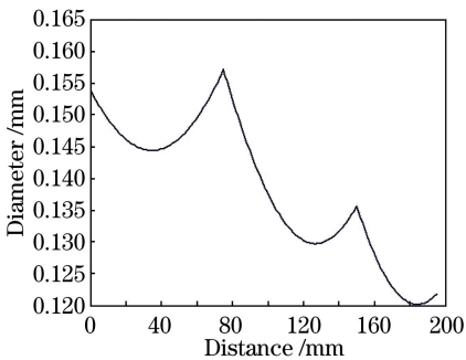
图 3 谐振腔内各位置处光斑直径
