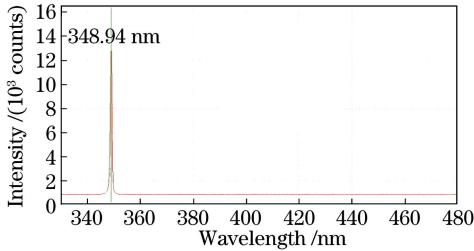
图 5 348.9 nm 紫外光的光谱
