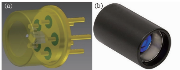
图 7 (a) 多波长激光二极管及(b) 其准直镜筒 三维效果图
