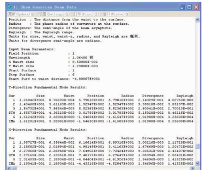
图5 1064 nm 离轴高斯光束的光路仿真结果
