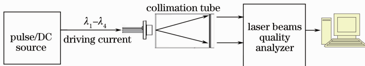
图 8 光束平行性验证实验原理图
