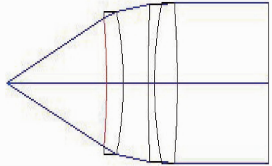
图4 准直光学系统的初始光路
