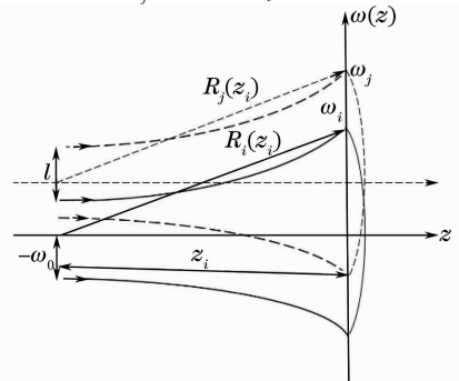
图 3 离轴高斯光束波面变化示意图
