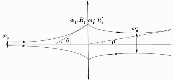
图 2 高斯光束传播和经过一次变换的原理图
