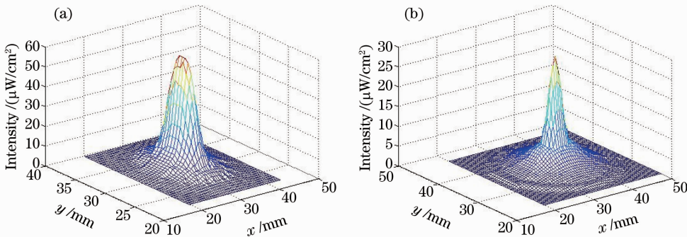
图 9 1064 nm(脉冲/单模)激光束腰光斑三维光强分布图。(a) 脉冲激光光斑; (b) 单模激光光斑
