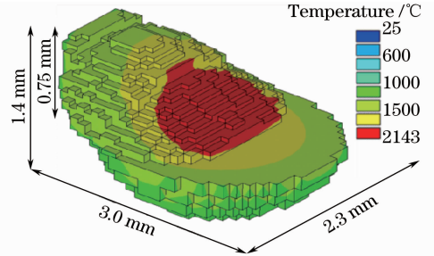
图7 根据温度场计算结果捕捉到的三维熔池形态
