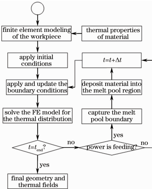
图 4 温度场及熔覆层几何形貌计算流程
