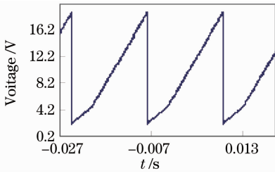
图 2 失真的锯齿波驱动信号
