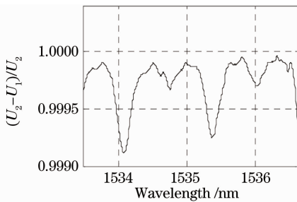
图 6 体积分数为 6.4 \times 10^{-5} 的乙炔气体多个吸收峰谱线图
