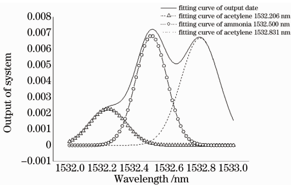
图 10 氨气乙炔吸收峰的混叠和 Origin 下的洛伦兹拟合示意图
