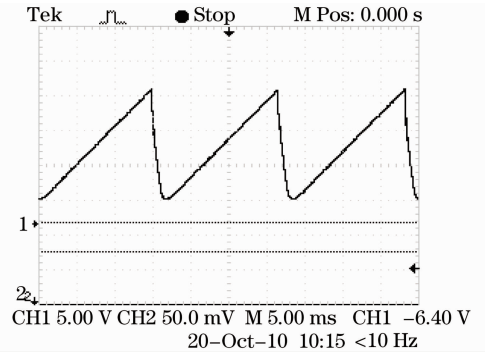
图 4 经过补偿后的锯齿波
