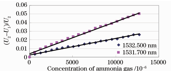
图 9 单一氨气气体定标结果
