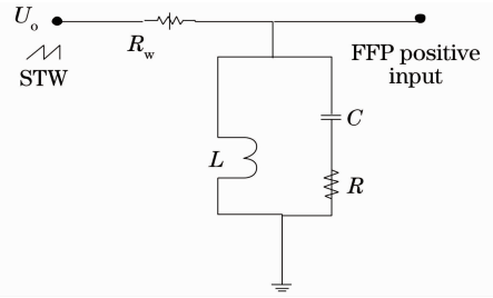
图 3 可调谐 F-P 滤波器的内部等效电路及补偿电路图
