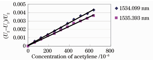
图 8 单一乙炔气体定标结果
