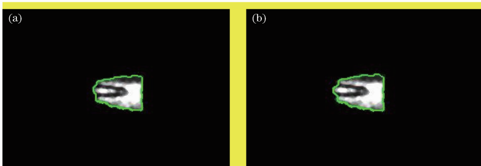
图5 激光(a)和日光灯(b)照明下经二值形态学方法提取的目标边界
