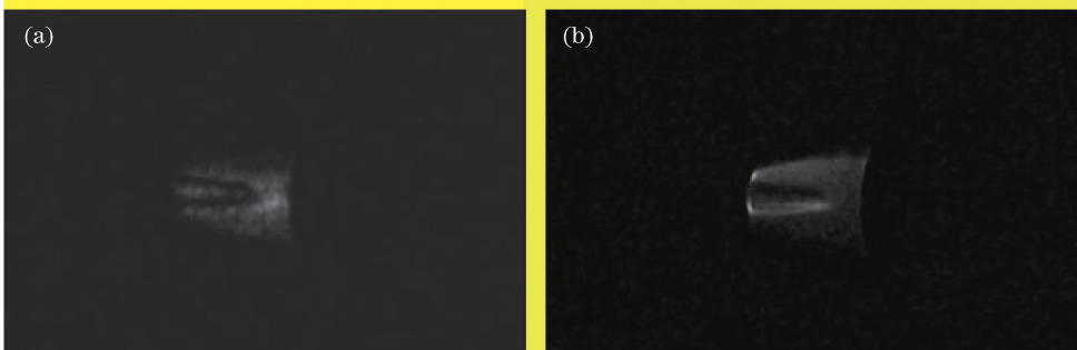
图 1 目标在激光(a)和日光灯(b)照明下的图像对比
