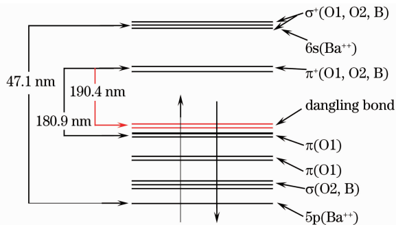
图 1 (\text{B}_3\text{O}_6)^{3-} 基团的能级结构
