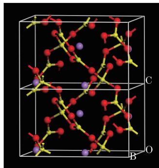
图 2 LBO 晶体的空间结构
