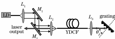
图 1 可调谐掺镱双包层光纤激光器示意图
