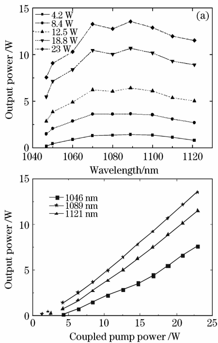
图3 (a) 不同入纤抽运功率时输出功率随调谐波长的变化;(b) 不同调谐波长处的输出功率随入纤抽运功率变化的特性曲线
