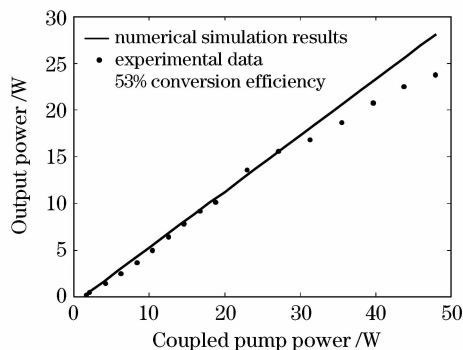
图5 调谐波长为1089 nm时的输出功率特性曲线 Fig. 5 Output power versus input pump power at 1089 nm
