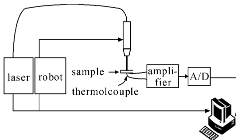
图 1 激光吸收率实验简易装置图
