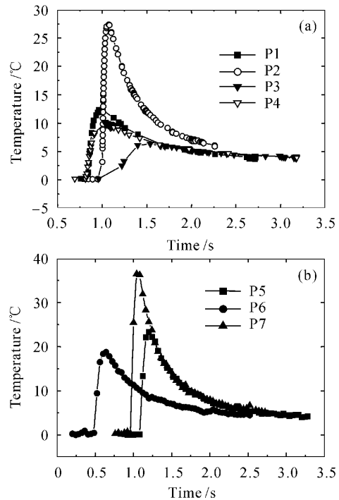
图 5 对应不同输入点的实验温度响应曲线
