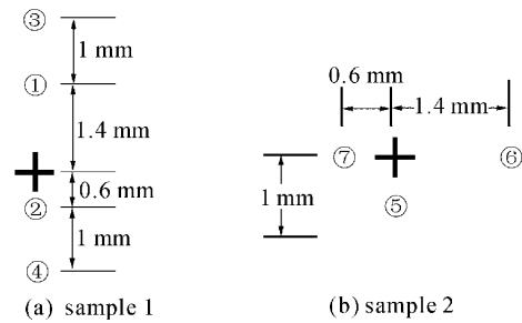
图 3 激光输入点分布图
