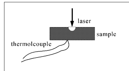
图 2 激光吸收率实验方案图
