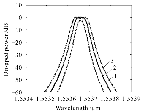
图 4 环间耦合系数对下话路滤波平坦度的影响
