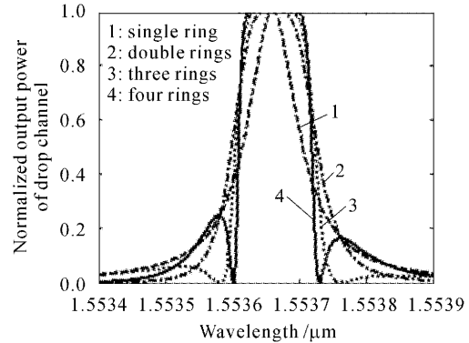
图 3 环型谐振腔个数对下话路滤波性能的影响
