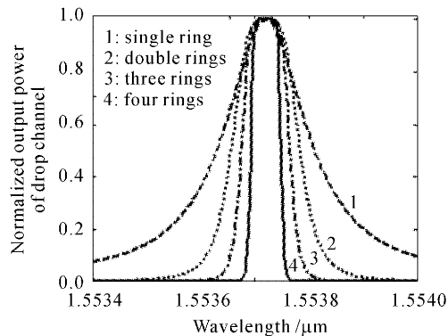
图 5 环型谐振腔个数对下话路滤波性能的影响
