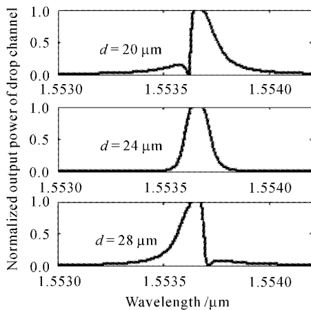
图 2 环间距对下话路滤波性能的影响
