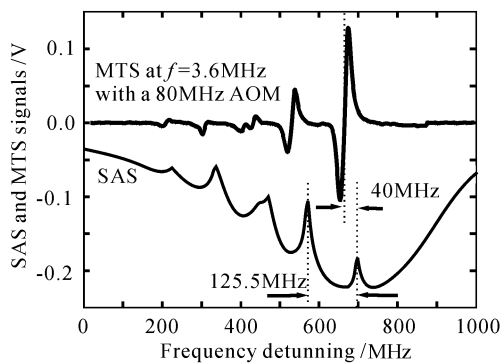
图 2 上方曲线(MTS)为铯原子 6^2S_{1/2} F=4 \rightarrow 6^2P_{3/2} F'=3,4,5 跃迁典型的调制转移光谱,抽运光路中的声光调制器工作在 80 MHz,其正弦调制频率为 3.6 MHz。下方曲线(SAS)为相应的饱和吸收光谱。相对于饱和吸收光谱而言,调制转移光谱红移了 40 MHz,正好是声光调制器工作频率的一半。曲线中的 6 个分量从左到右分别对应于铯原子 F=4 \rightarrow F'=3 跃迁, F=4 \rightarrow F'=3,4 交叉线, F=4 \rightarrow F'=4 跃迁, F=4 \rightarrow F'=3 和 5 交叉线, F=4 \rightarrow F'=4 和 5 交叉线,和 F=4 \rightarrow F'=5 跃迁
