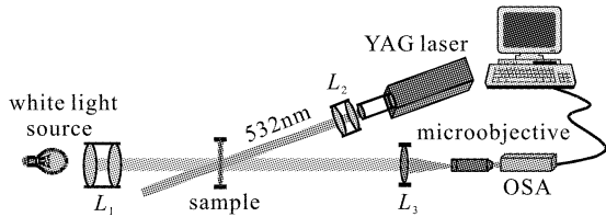
图 2 BR 膜静态光谱测试的实验装置图
