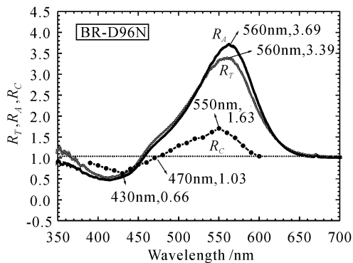
图 8 随读出光波长变化的 R_A 与 R_T 曲线和图像对比度 R_C 线
