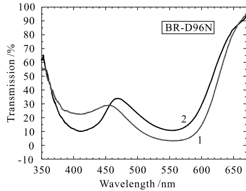
图 4 BR 薄膜经 532 nm 激发光作用前(曲线 1)和后(曲线 2)的透射光谱
