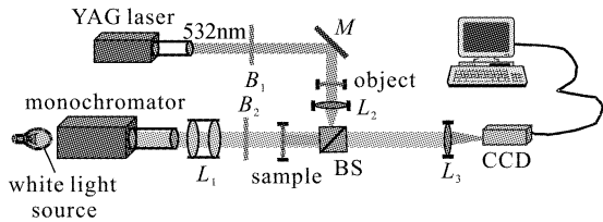
图 3 BR 膜记录图像的实验装置图
