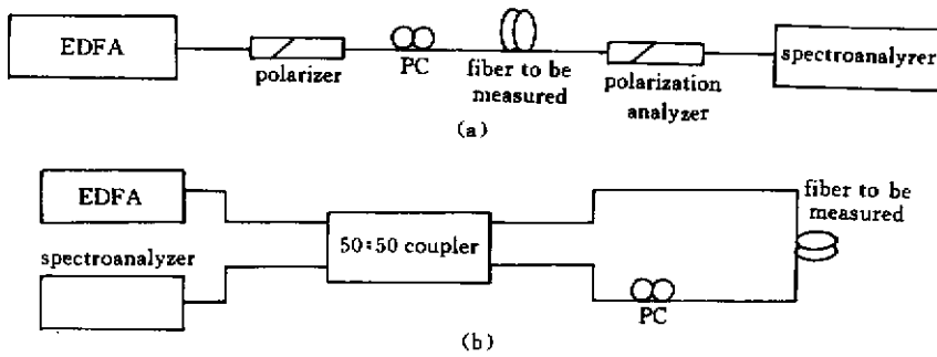
图 1 固定分析法(a)和 Sagnac 干涉法(b)测量原理方框图
