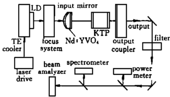
图 1 LD 抽运 Nd:YVO 4 /KTP 腔内倍频绿光激光器示意图
