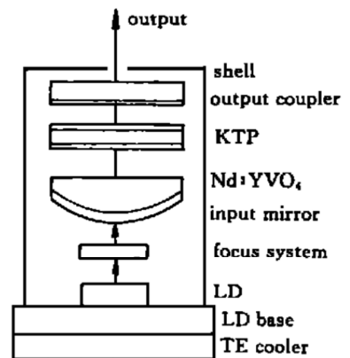
图 2 LD 抽运的高性能微型绿光激光器结构图
