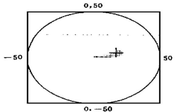
图4 输出光束 24 h 的方向稳定性测试图 Fig.4 Direction stability of the output beam in 24 hours
