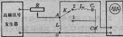
图4 串并联法测量分布电感线路图
