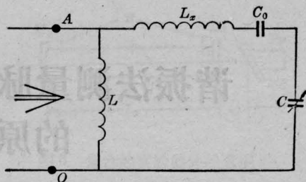
图2 串并联谐振电路图
